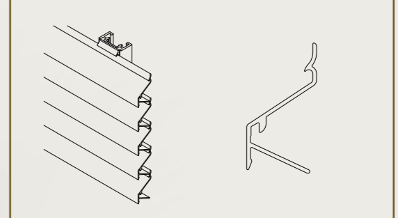
L.033CL – Geschlossenes Profil
